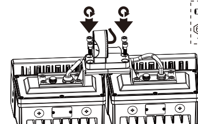
Double module
