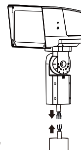
Single Module
